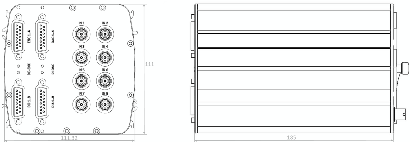
Die Abbildung zeigt ein CS Gerät in Standard-Gebrauchslage.
