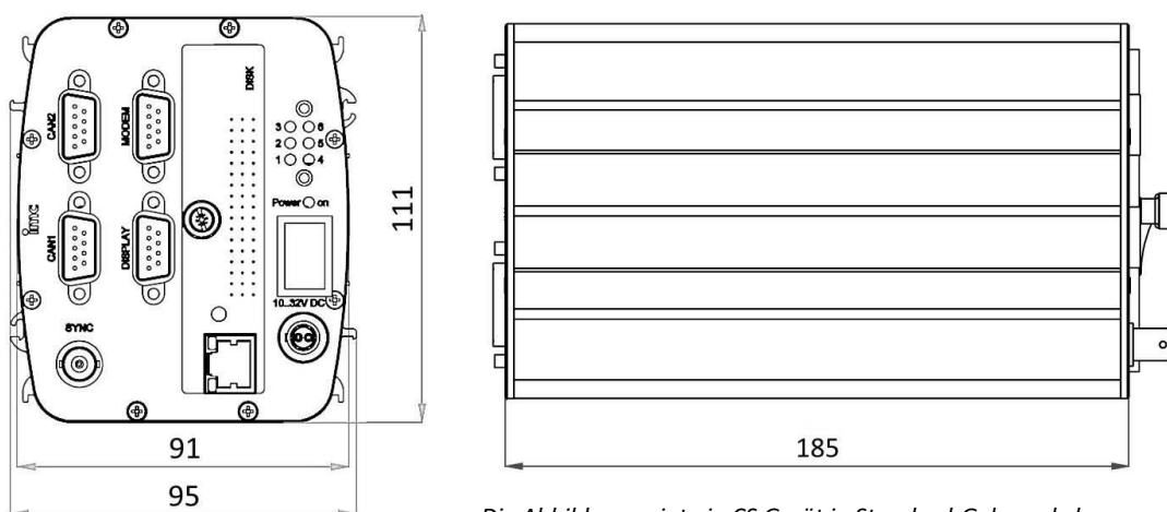
Die Abbildung zeigt ein CS Gerät in Standard-Gebrauchslage.
