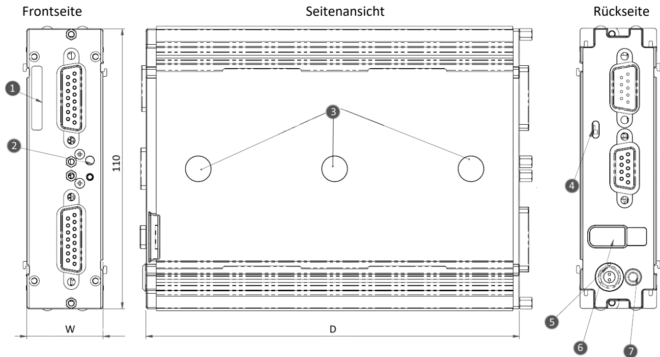
Die Abbildung zeigt ein Modul in Standard-Gebrauchslage: Gehäusetyyp L0 mit einer Breite (W) von 30 mm.
