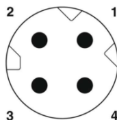
M8-Stecker, D-kodiert (Sicht auf die Stifte)
