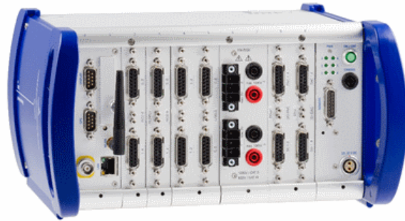
imc CRONOScompact: Tragegehäuse CRC-400-08
