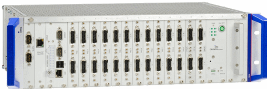
imc CRONOScompact: 19" Baugruppenträger CRC-400-AC-RACK
