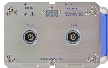
CRFX/HISO-8-T-2L
