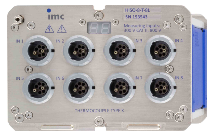
CRFX/HISO-8-T-8L
