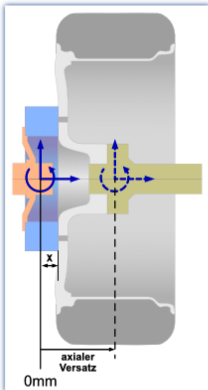
Axialer Versatz
