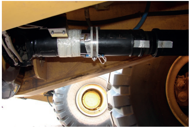
Messung des Drehmoments an Muldenkipper
