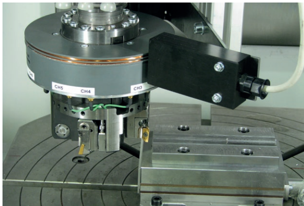
Kraftmessung an Fräsmaschine
