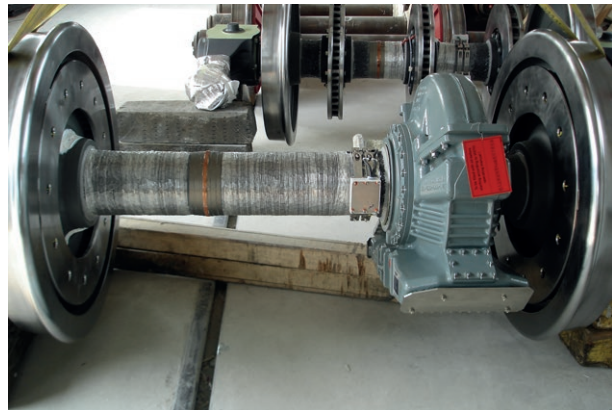
Temperaturmessung an Bahn-Bremsscheibe
