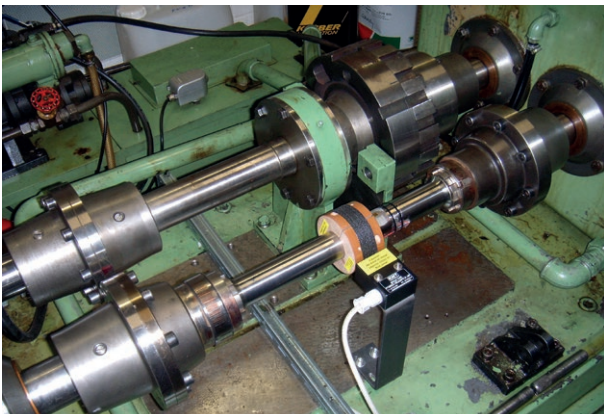
Messung des Drehmoments am Getriebe-Prüfstand
