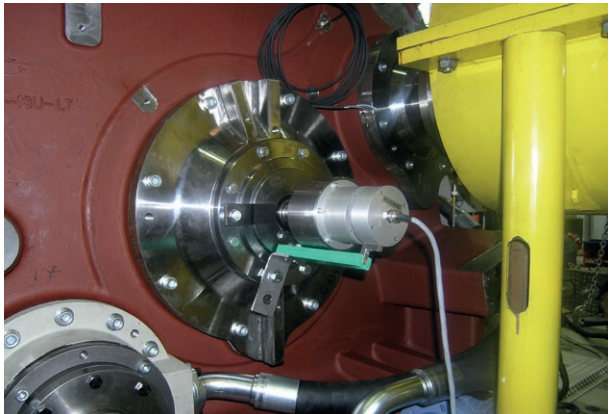
Kraftmessung bei großem Getriebe-Prüfstand
