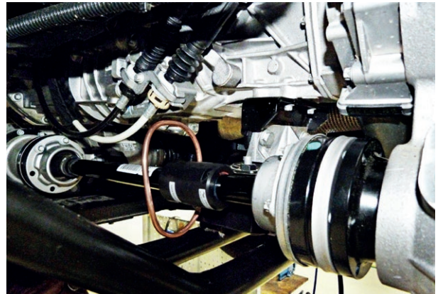
Drehmomentmessung an Antriebswelle mit D x
