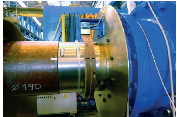
Drehmomentmessung an Antriebswelle
