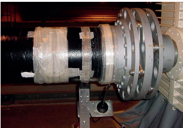
Drehmomentmessung an Schiffs-Antriebswelle
